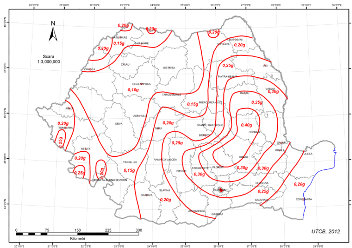
Figura 8: Zonarea valorilor de vârf ale accelerației terenului pentru proiectare a_g cu IMR = 225 ani (20% probabilitate de depășire în 50 de ani)
