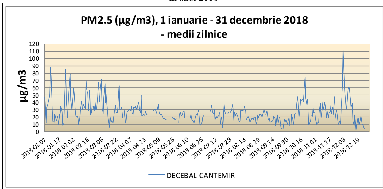
Figura I.3.3.3. Valori medii zilnice pentru particule în suspensie PM 2,5 determinate gravimetric în anul 2018
