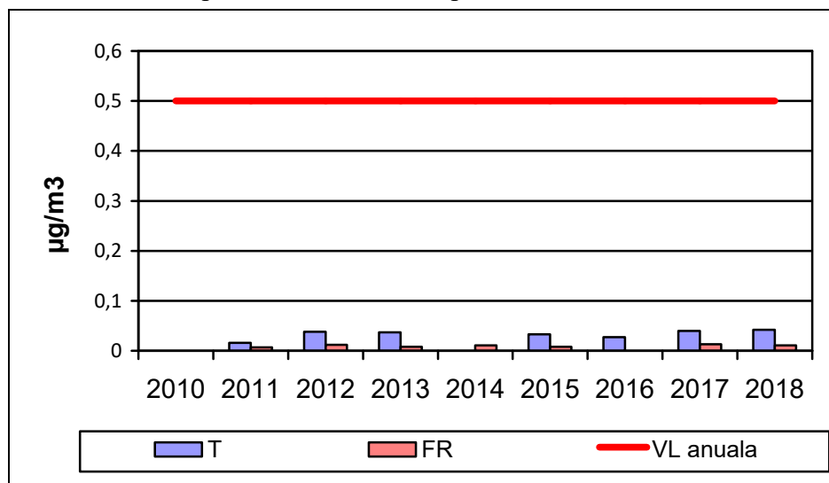
Figura I.I.6. Pb gravimetric determinat din fracția PM10 – Evoluția concentrațiilor medii anuale înregistrate la stațiile de monitorizare în raport cu VL anuală, în perioada 2010 – 2018
