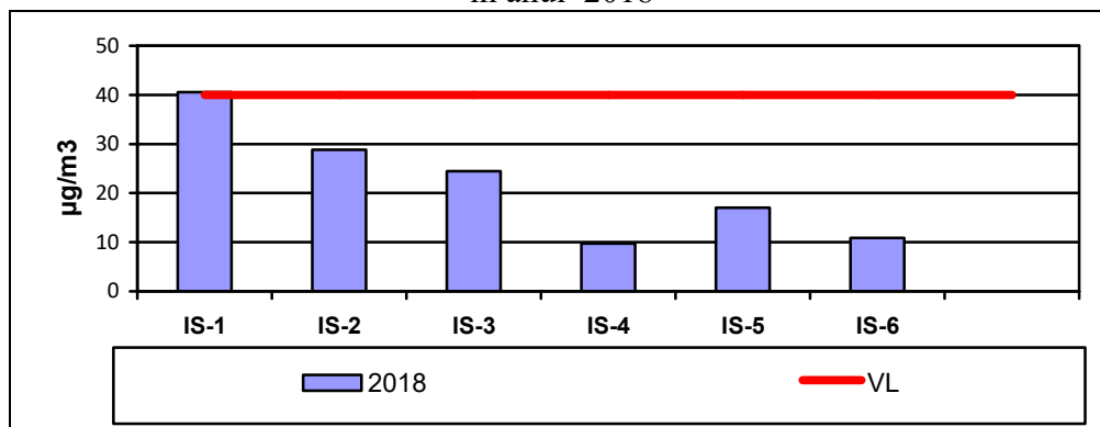
Figura I.3.1.2. NO 2 - Concentrațiile medii anuale înregistrate la stațiile de monitorizare, în anul 2018
