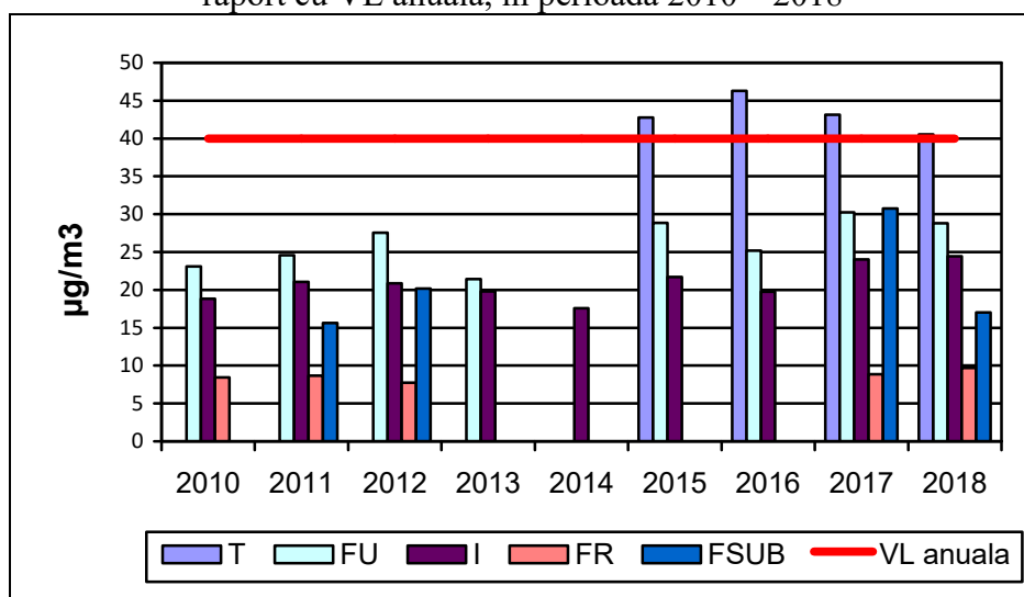
Figura II.1. NO 2 – Evoluția concentrațiilor medii anuale înregistrate la stațiile de monitorizare în raport cu VL anuală, în perioada 2010 – 2018
