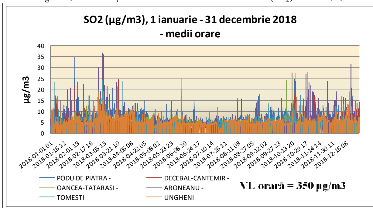
Figura I.3.2.1. Variația mediilor orare ale dioxidului de sulf (SO 2 ) în anul 2018
