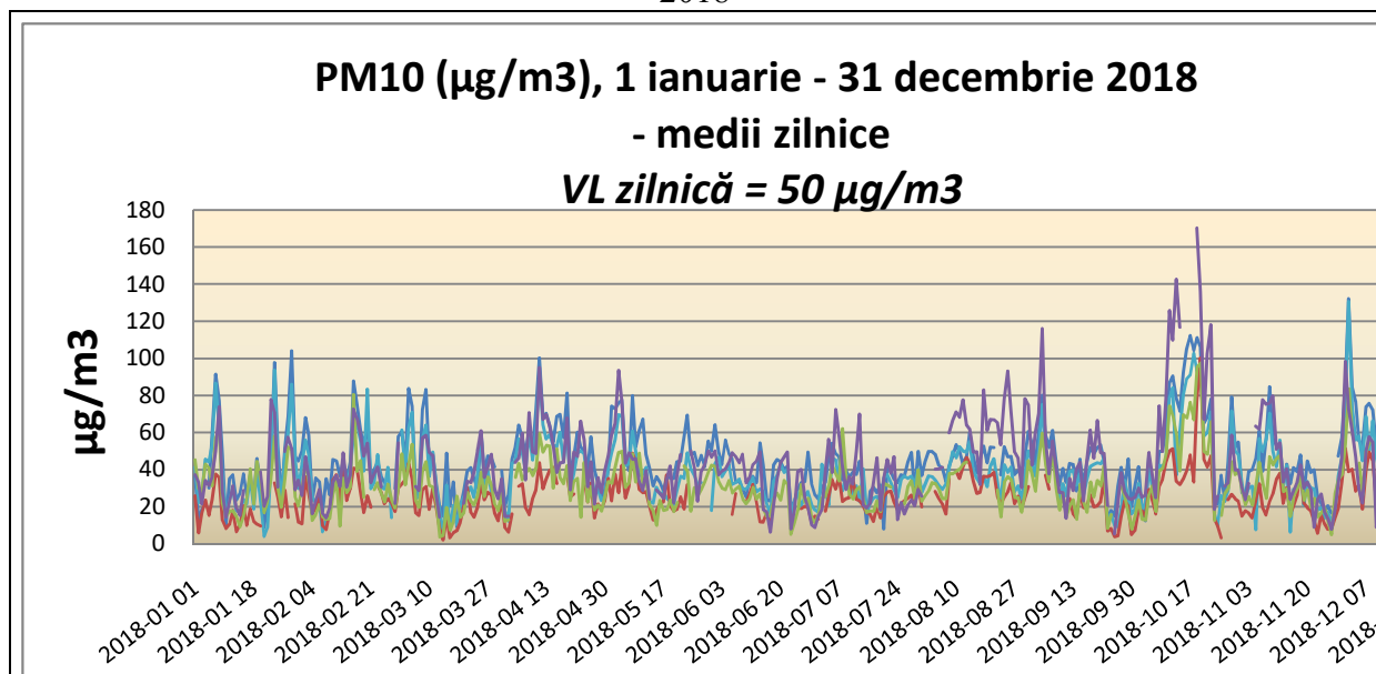
Figura I.3.3.2. Valori medii zilnice particule in suspensie PM10 determinate gravimetric în anul 2018
