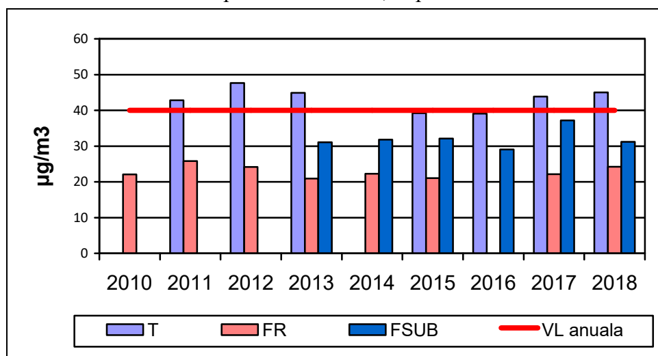
Figura II.3. PM 10 gravimetric – Evoluția concentrațiilor medii anuale înregistrate la stațiile de monitorizare în raport cu VL anuală, în perioada 2010 – 2018
