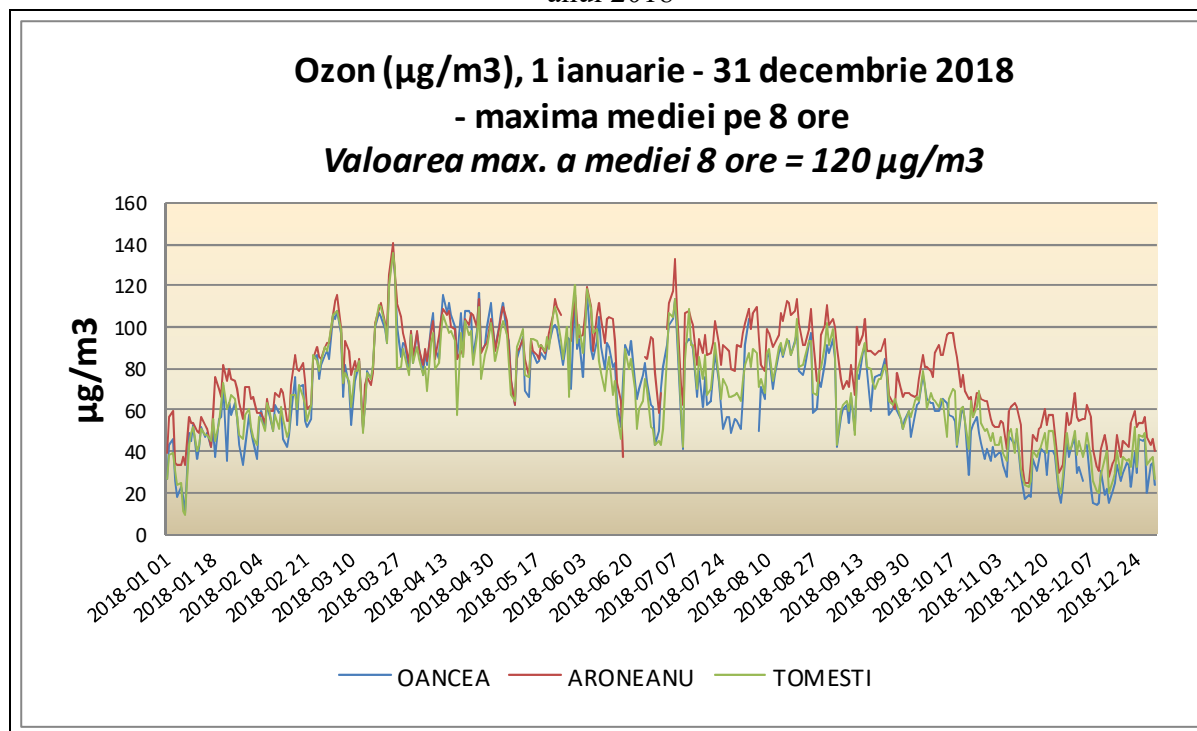
Figura I.3.8.2. Variația valorilor maxime zilnice a mediilor pe 8 ore a concentrației de ozon în anul 2018
