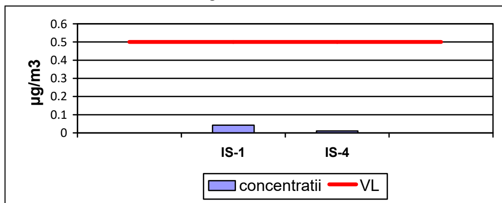
Figura I.3.4.1. Pb gravimetric determinat din fracția PM10 – Concentrațiile medii anuale înregistrate la stațiile de monitorizare, în anul 2018
