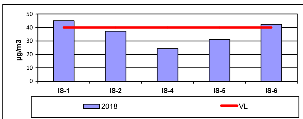
Figura I.3.3.1. PM10 gravimetric - Concentrațiile medii anuale înregistrate la stațiile de monitorizare din județul Iași, în anul 2018
