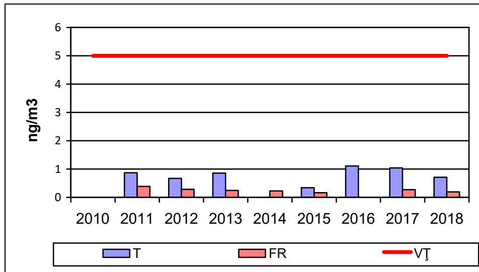
Figura I.I.7. Cd gravimetric determinat din fracția PM10 – Evoluția concentrațiilor medii anuale înregistrate la stațiile de monitorizare în raport cu VL anuală, în perioada 2010 – 2018
