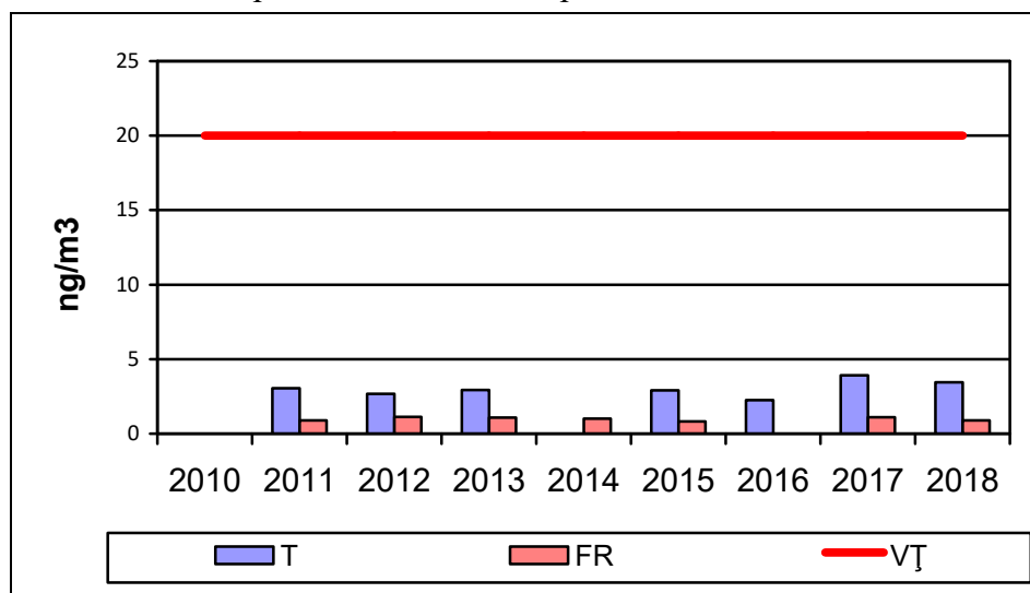
Figura I.I.8. Ni gravimetric determinat din fracția PM10 – Evoluția concentrațiilor medii anuale înregistrate la stațiile de monitorizare în raport cu VL anuală, în perioada 2010 – 2018
