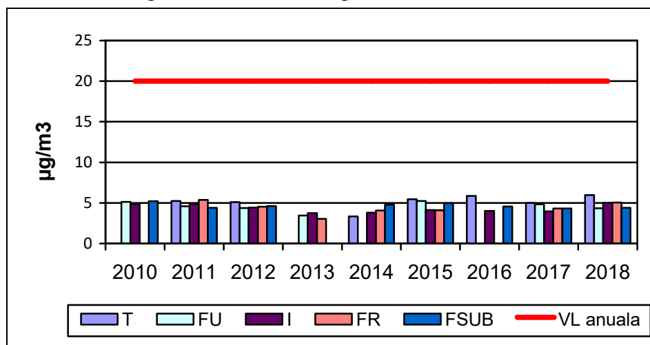
Figura II.2. SO 2 – Evoluția concentrațiilor medii anuale înregistrate la stațiile de monitorizare în raport cu VL anuală, în perioada 2010 – 2018
