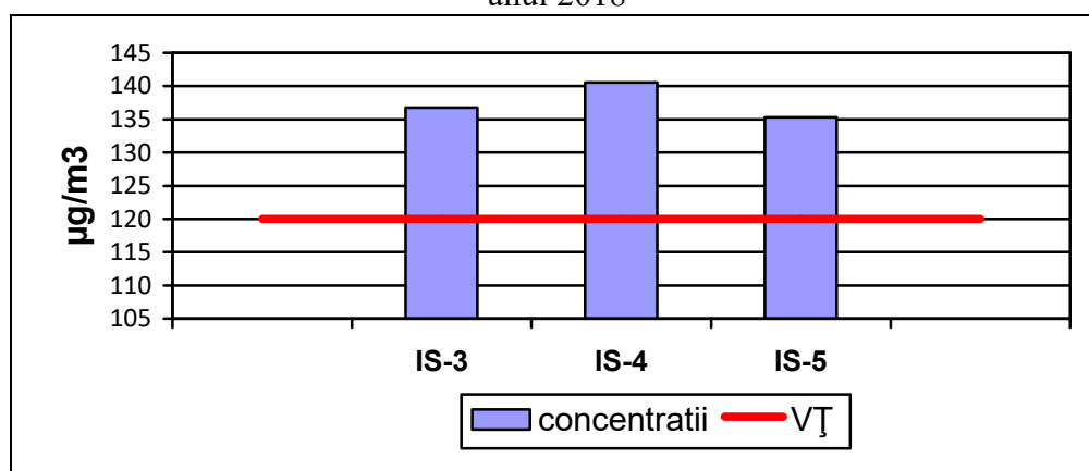
Figura I.3.8.1. Ozon – Maxima zilnică mediei pe 8 ore, înregistrate la stațiile de monitorizare, în anul 2018
