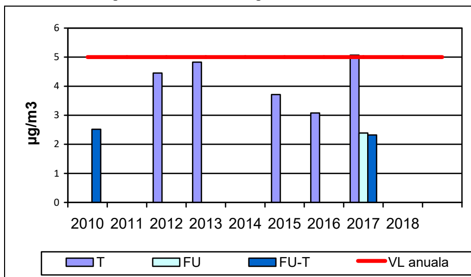
Figura I.I.5. C 6 H 6 – Evoluția concentrațiilor medii anuale înregistrate la stațiile de monitorizare în raport cu VL anuală, în perioada 2010 – 2018
