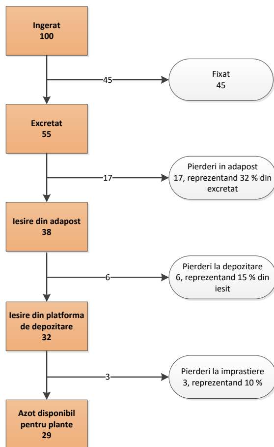
Diagrama fluxului de azot în cazul gestionării dejectiilor de la pui crescuți la sol, pe așternut
